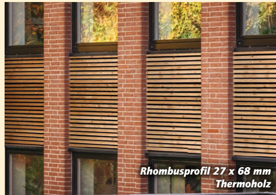
Rhombusprofil 27 x 68 mm Thermoholz
