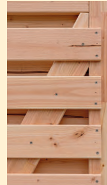
Borkum Tür, Verschraubung, Innen- bzw. Außenansicht
