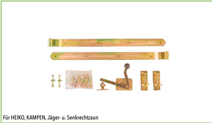
Für HEIKO, KAMPEN, Jäger- u. Senkrechtzaun
