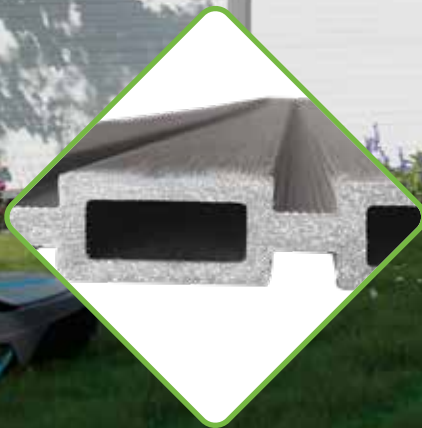
WAREN weiß mit silberfarbenen Aluminium-Steckzaunpfosten und Aluminium-Abschlussleisten
